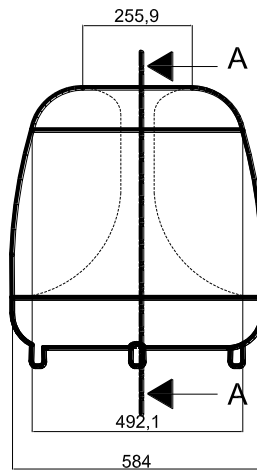
ΠΡΟΟΨΗ
