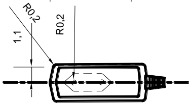
ΠΡΟΟΨΗ
