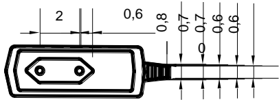
ΚΑΤΟΨΗ
