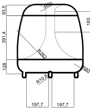
ΑΡΙΣΤΕΡΗ ΟΨΗ
