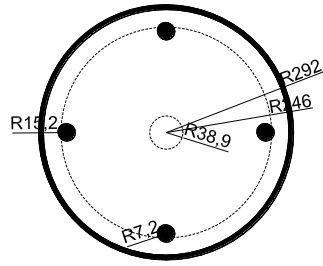
ΚΑΤΟΨΗ
